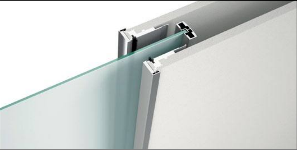
Porta scorrevole a scomparsa con stipite Free / Pocket sliding door with Free jamb
